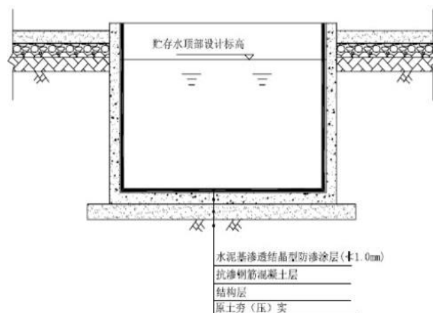
图 5.1-5 事故处理池防渗示意图
