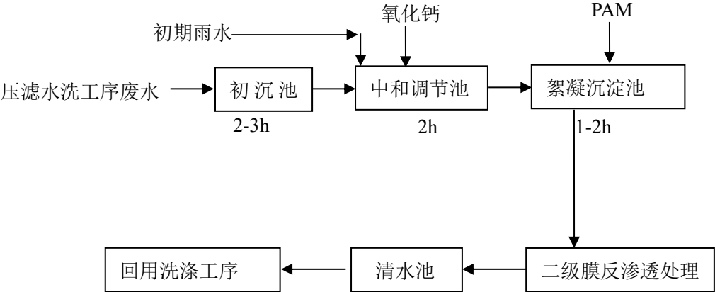
图 5.1-1 废水处理工艺流程图
