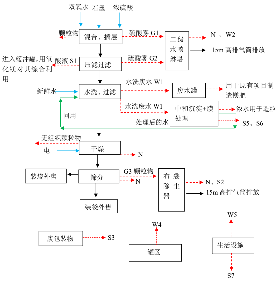
图 2.2-3 直接用双氧水生产工艺流程图
