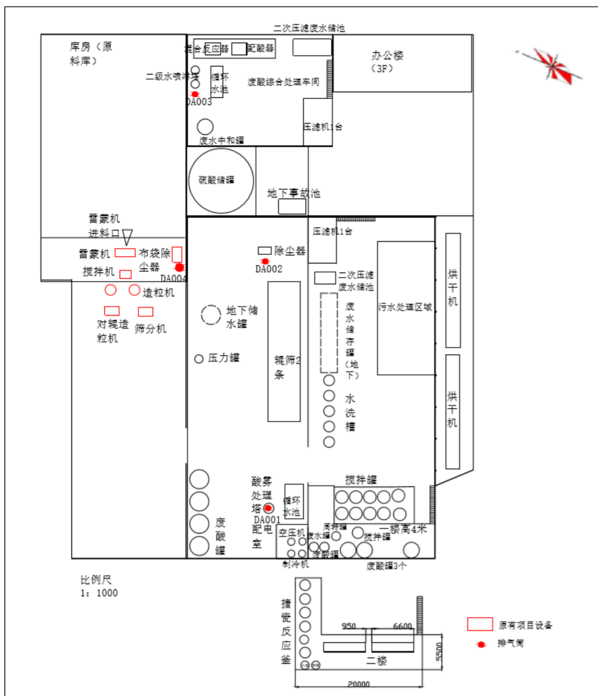
图2.2-1 厂区及车间设备平面布置图
